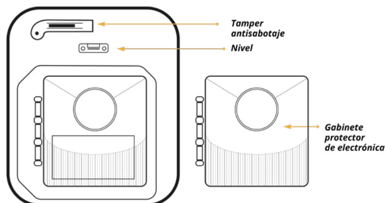
Vista Interior de la Sirena
