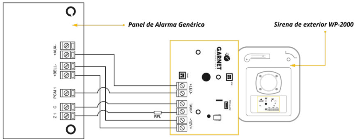
Esquema de conexión
