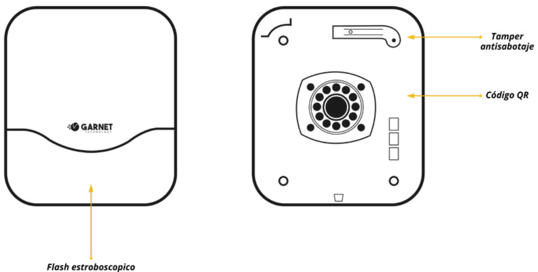
Vista Interior de la Sirena
