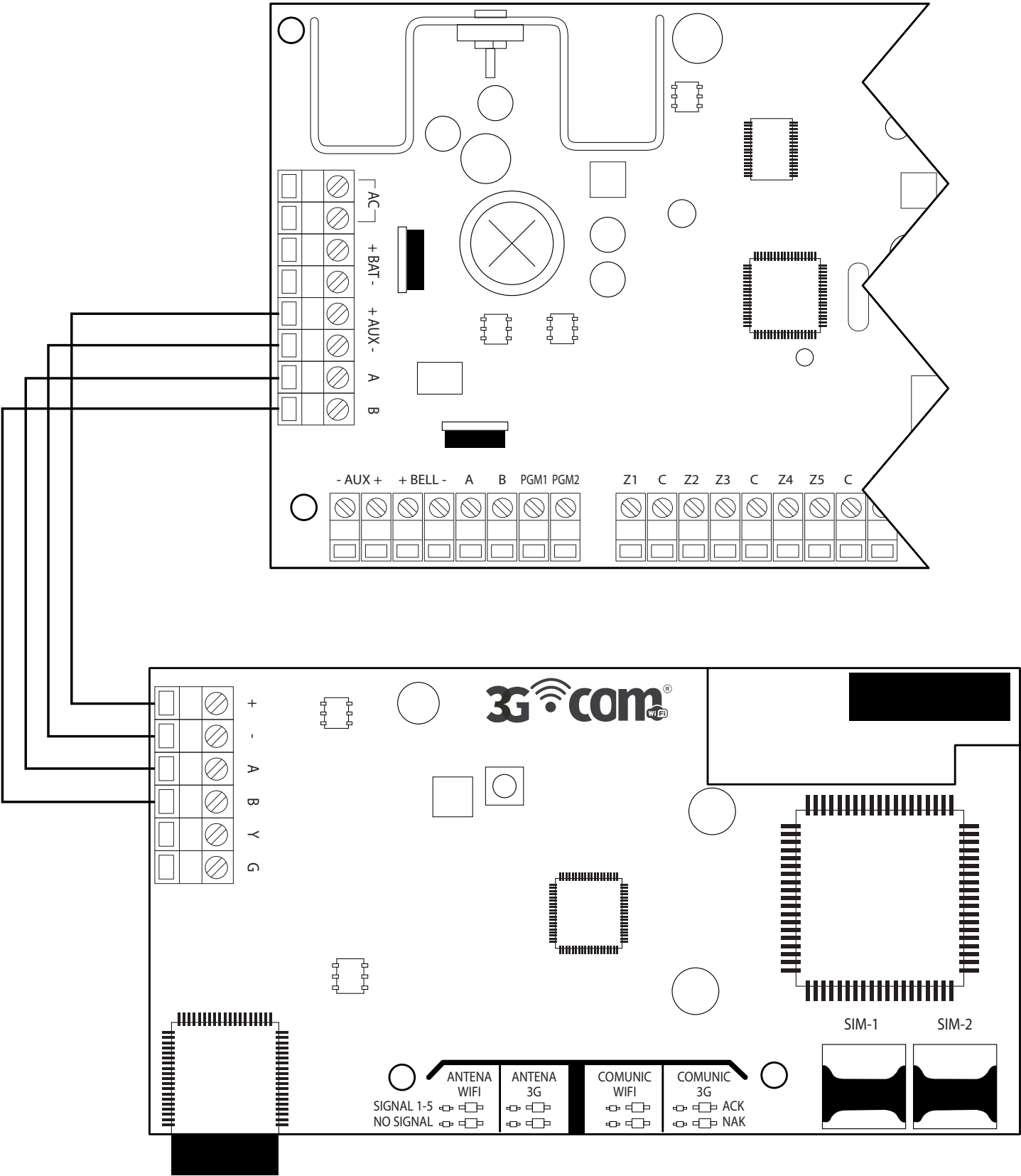
Conexionados: Figura 1 - Modo de operación BUS-C485:
